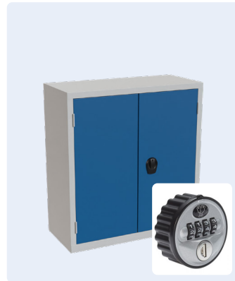
Artikelnr. 131V0011-218 MS-0.5 med 2 galv. hyllor och Eurolock kodlås Modell A099 Utvändigt mått mm: H:1075 B:1000 D:445 Karmmått i mm: H:945 B:920 D:425
