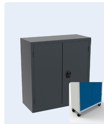
Artikelnr. 131V0011-S MS-0.5 med 2 galv. hyllor och 80 mm. hjul Utvändigt mått mm: H:1180 B:1000 D:445 Karmmått i mm: H:945 B:920 D:425
